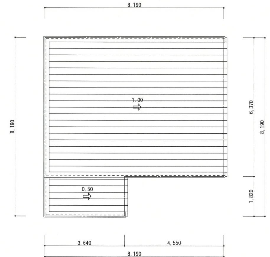
2階 屋根伏図 S:1/100
